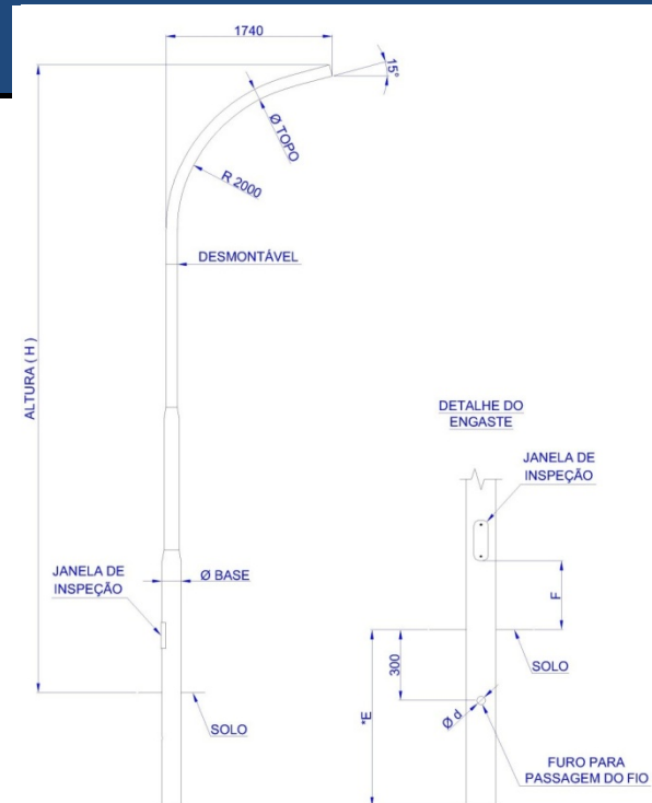
DESENHO TÉCNICO ILUSTRATIVO
