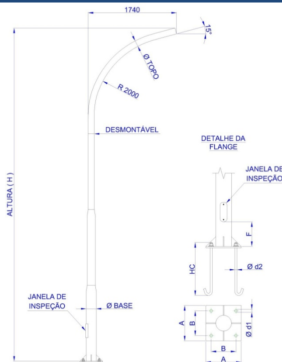
DESENHO TÉCNICO ILUSTRATIVO
